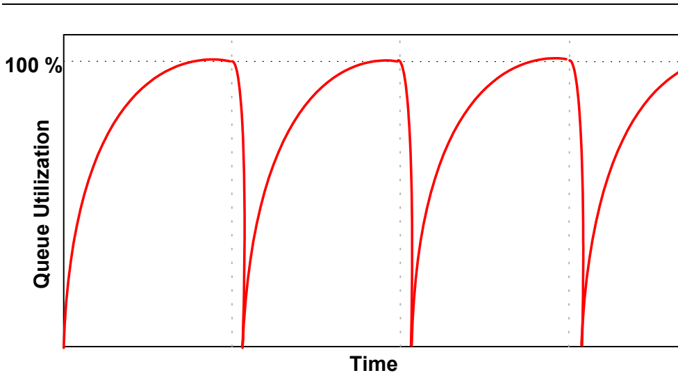
Abbildung 3.4: Queue-Auslastung beim Global-Synchronisation-Effekt
