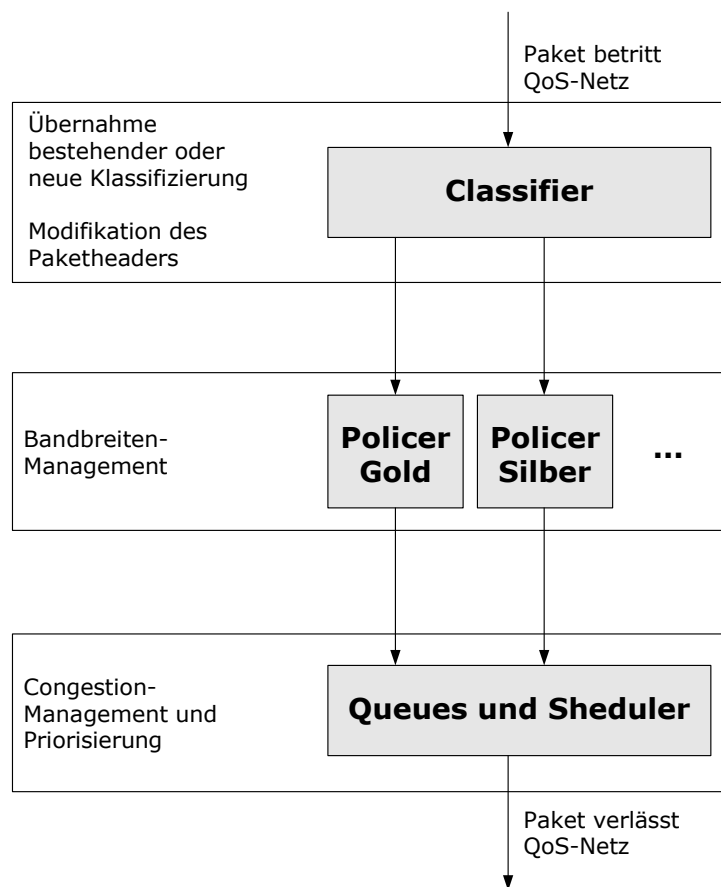
Abbildung 3.5: Ablaufschema des Differentiated-Service-Modells
