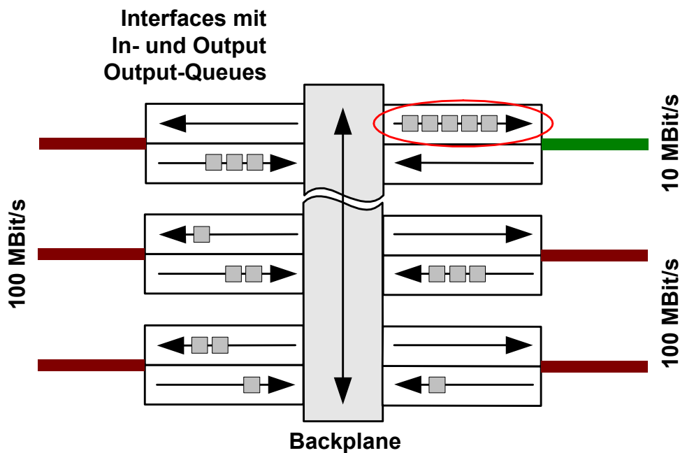
Abbildung 3.2: interne Struktur eines Switches, Überlauf eines Output-Puffers
