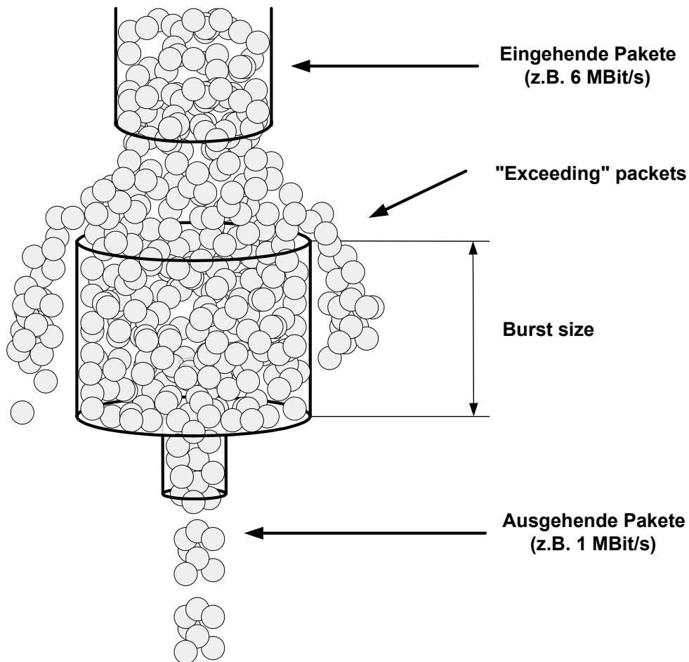
Abbildung 4.2: Bildliche Darstellung des Token-Bucket-Algorithmus zum Bandbreiten-Management
