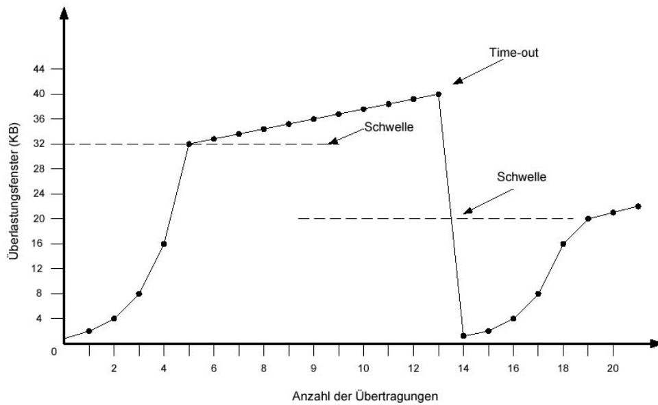
Abbildung 3.3: Überlastalgorithmen von TCP (Darstellung aus [Tan98])
